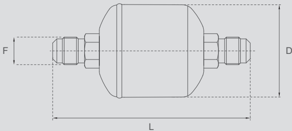
Dimensioni - Dimensions
